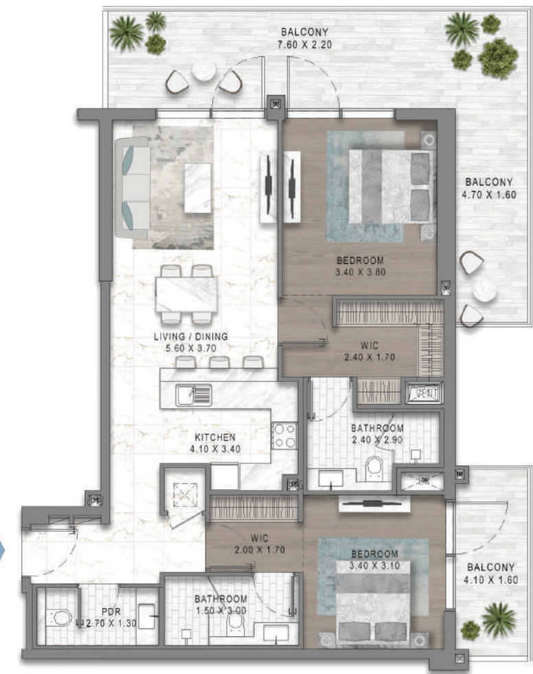
2BR - TYPE A3
