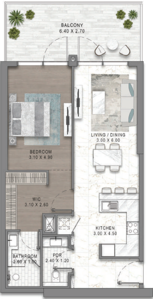
1BR - TYPE A2
