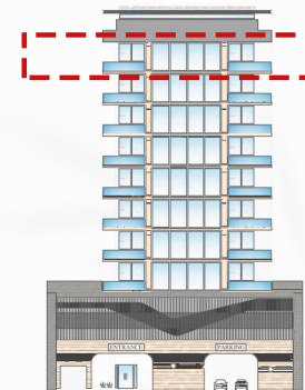
Key Elevation
